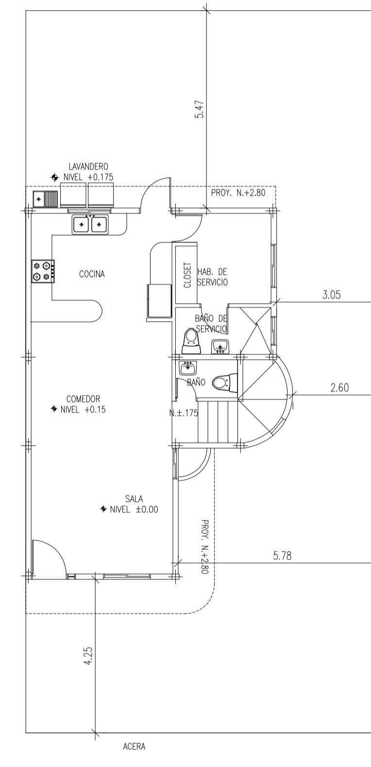
UBICACION TIPICA ESC: 1/100
