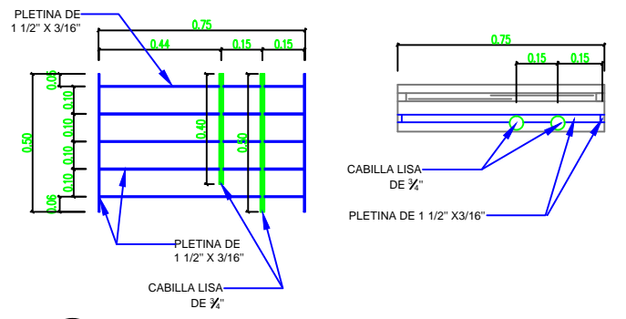
3 VENTANA TIPO V-3 Escala: 1:25
